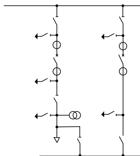
Двойная система сборных шин с обходным разъединителем
