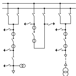
Полуторная схема соединения шин
