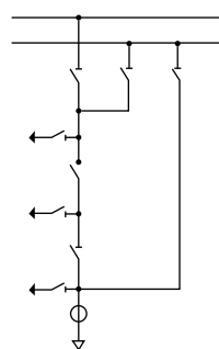
Двойная система сборных шин с обходным разъединителем
